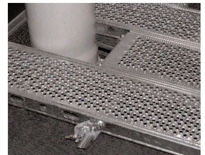
Apertura de huecos con plataformas T4
