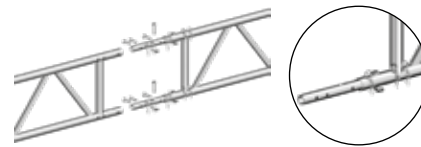
Posibilidad de conexión con grapa a viga ref. 4904
