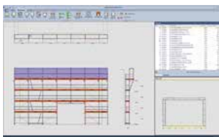
Andamio de fachada con vigas de celosía, ménsulas y rejillas de protección
