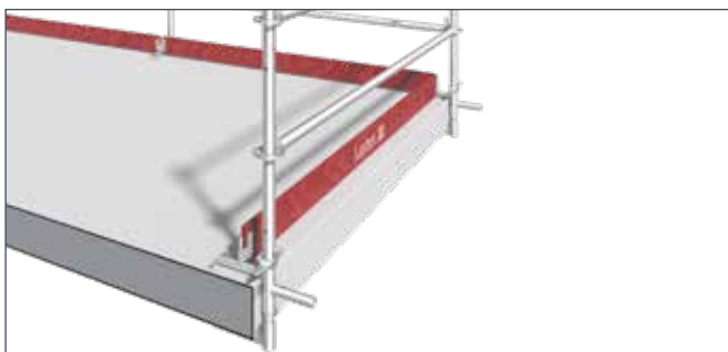
Ejemplo de aplicación de la mordaza para forjados.
